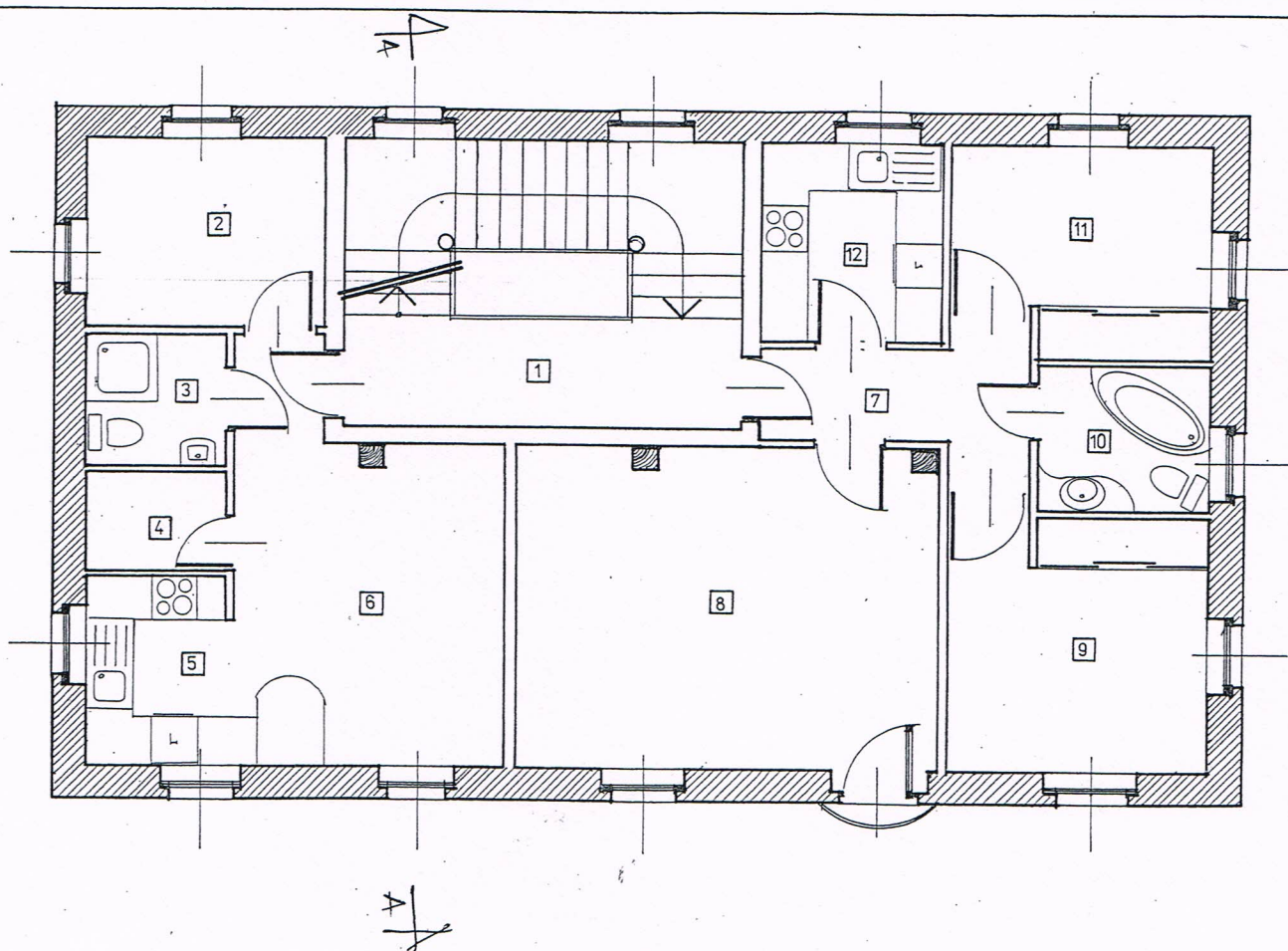
ASAPTACYA BUDYNKU SCINAWKA DŁN N°1 RZUT I i II PIĘTRA 1:100
