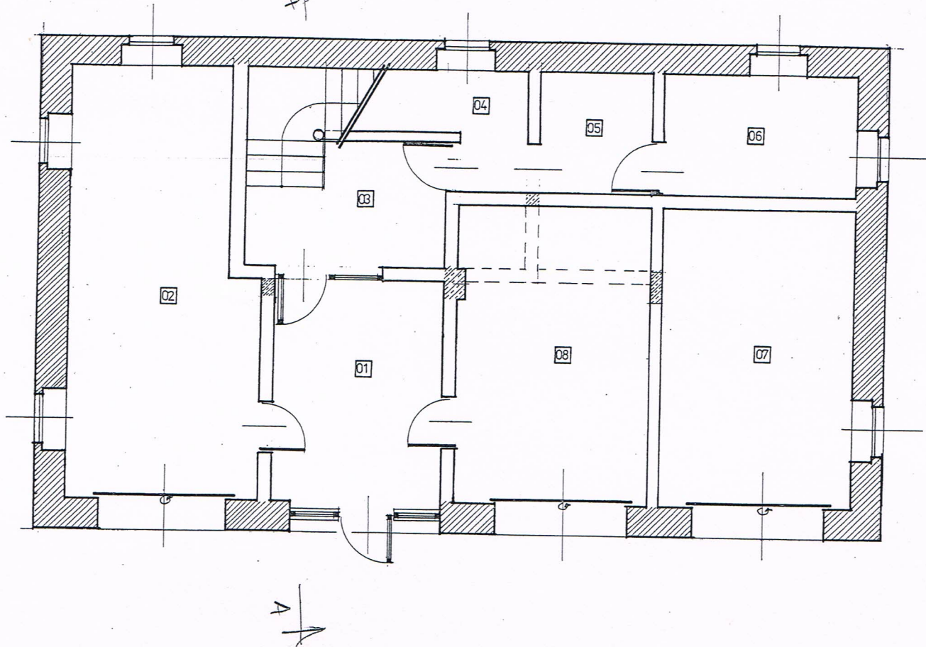
ASAPTACYA BUDYNKU SCINAWKA DŁN N°1 RZUT PARTERU 1:100
